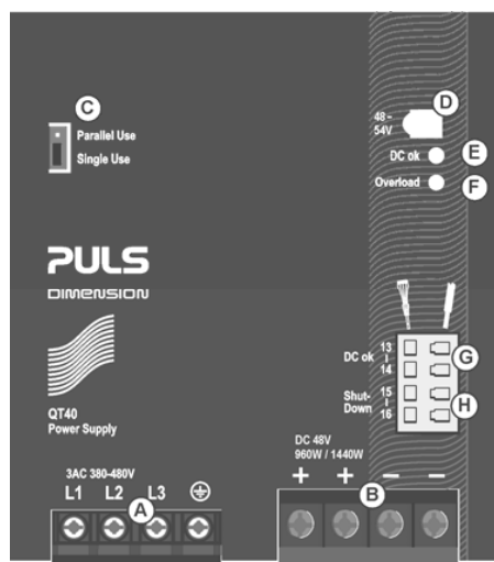
Fig. 15-1 Front side
