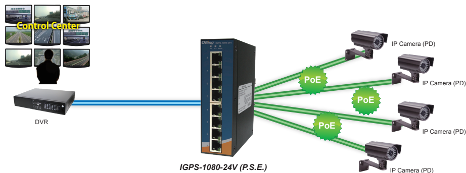
IGPS-1080-24V (P.S.E.)
